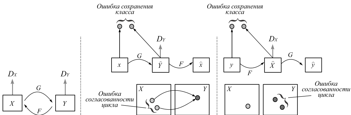
Рис. 1. Схема генерации изображений, улучшенных syclgan, с сохранением класса дорожного знака
